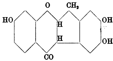
Brasilein
